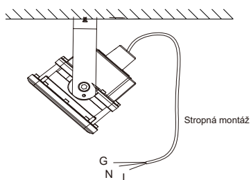
1-Stropná montáž
