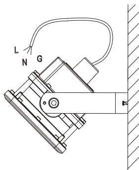
2-Nástenná montáž
